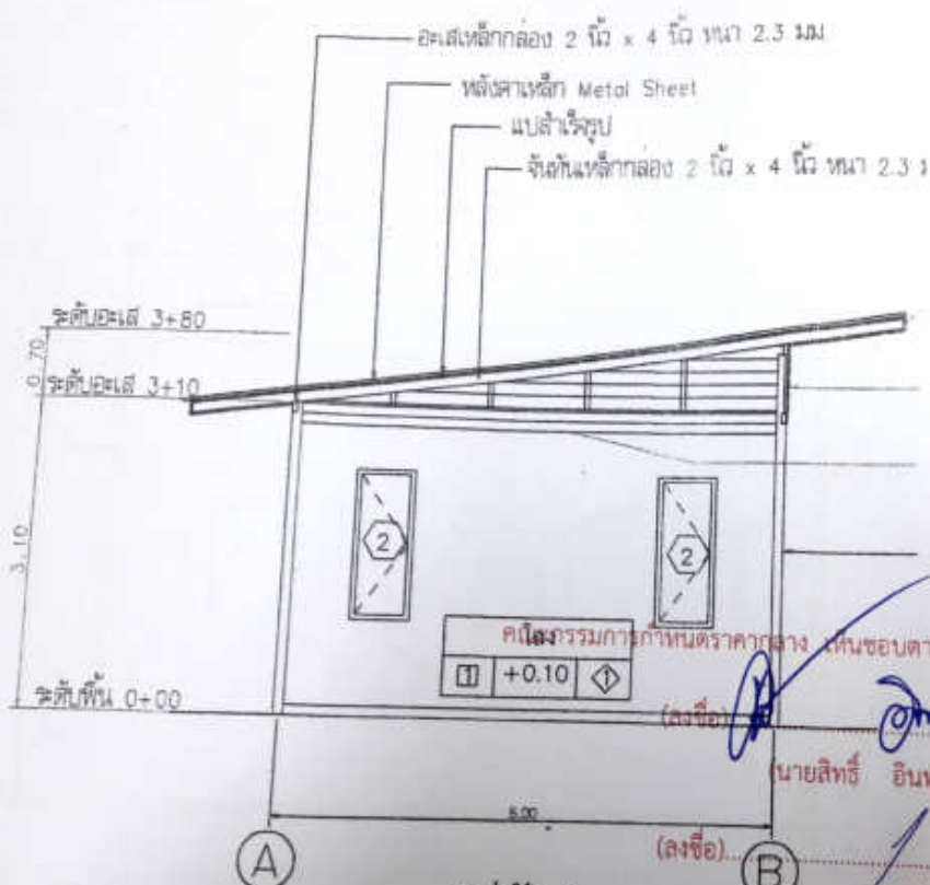
รูปตัด A มาตรฐาน 1:75
